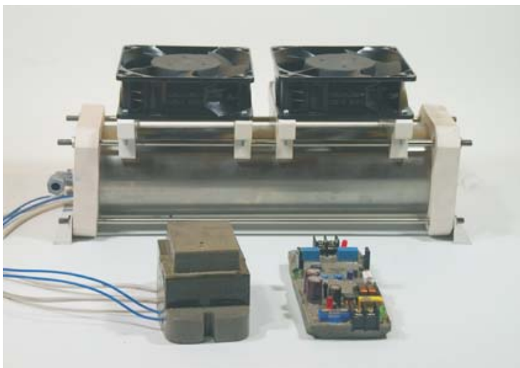
Conjunto Reactor 12T + Inverter + Transformador
